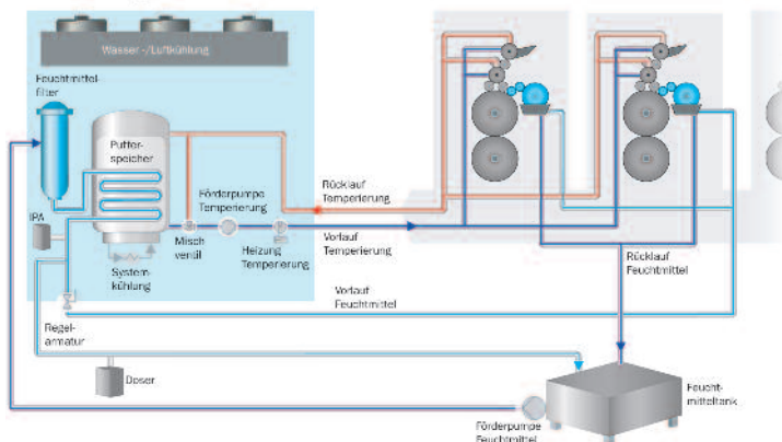
CT-EX-Fließdiagramm
